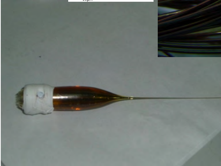
预制棒丝头
